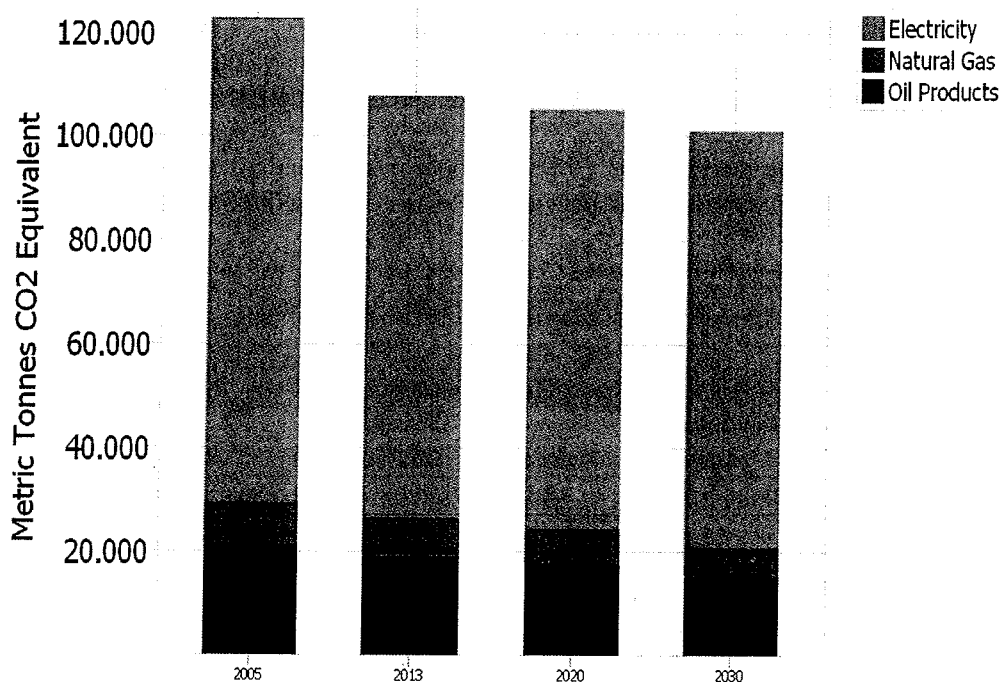
Figura 77: Emissioni per fonte nello scenario business-as-usual (ton. Eq.CO2)
