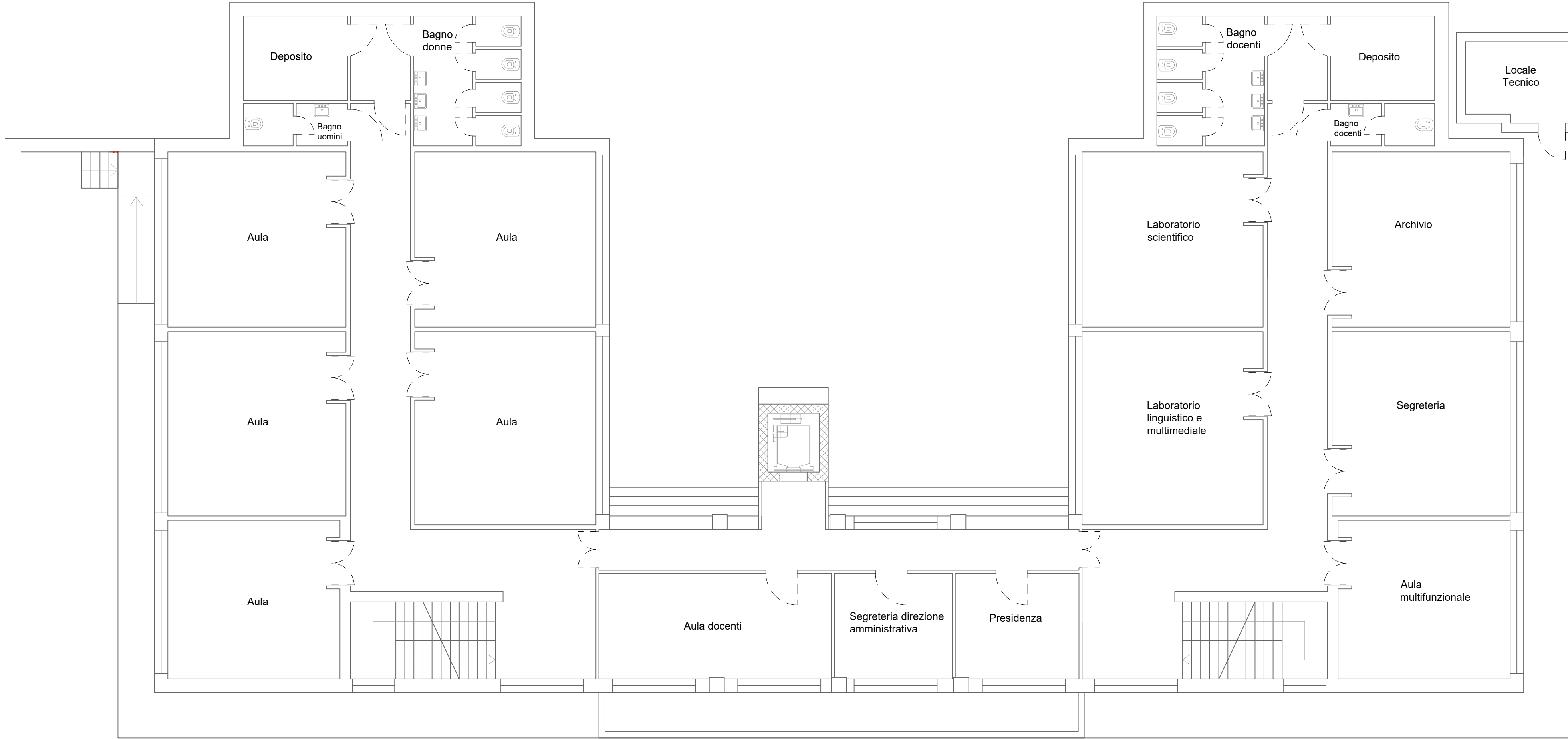
PIANO PRIMO
