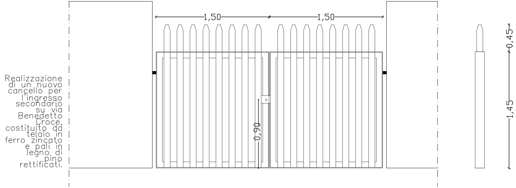
PARTICOLARE COSTRUTTIVO DI PROGETTO: CANCELLO scala 1:20
