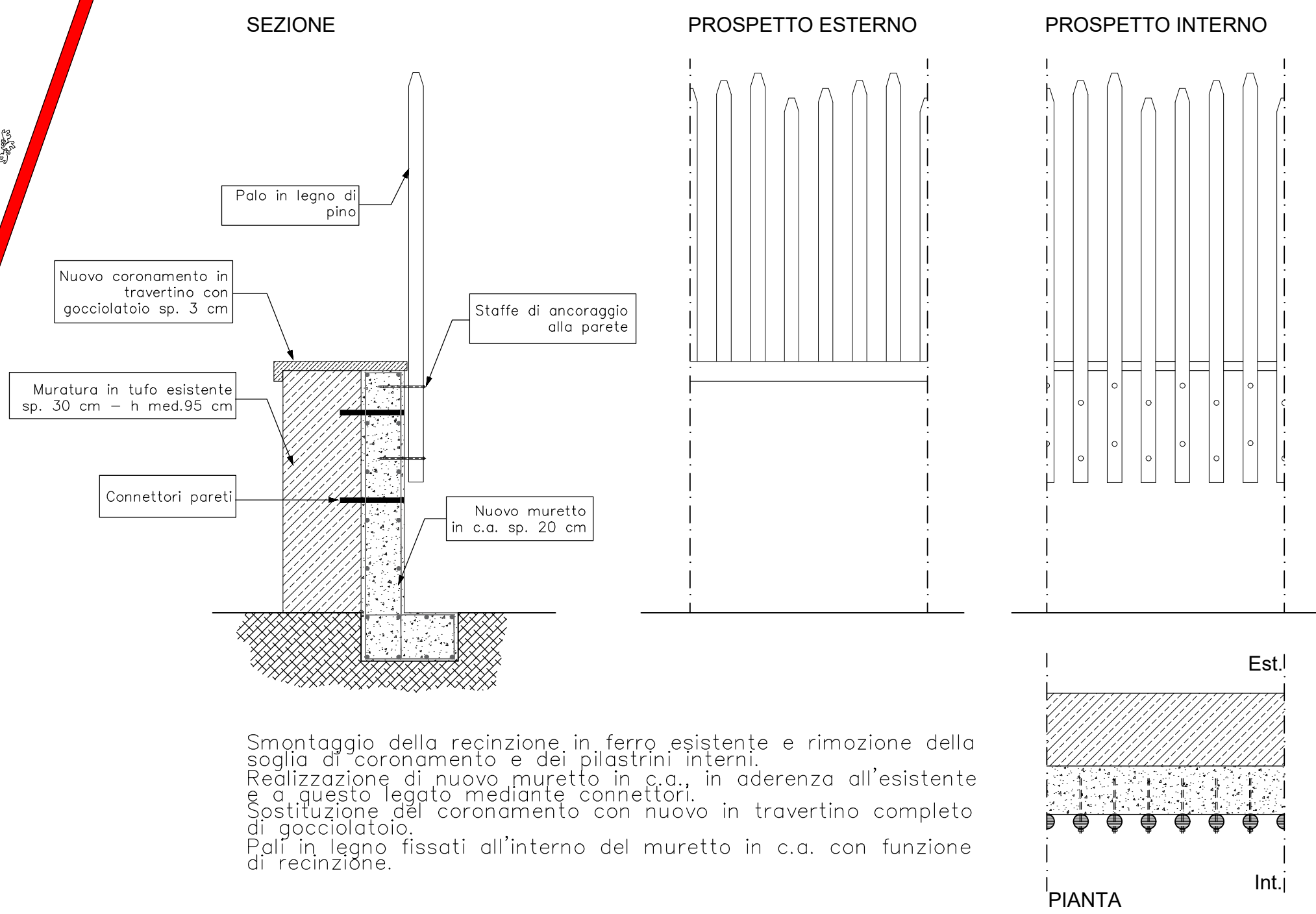
PARTICOLARE COSTRUTTIVO DI PROGETTO: RECINZIONE scala 1:20
