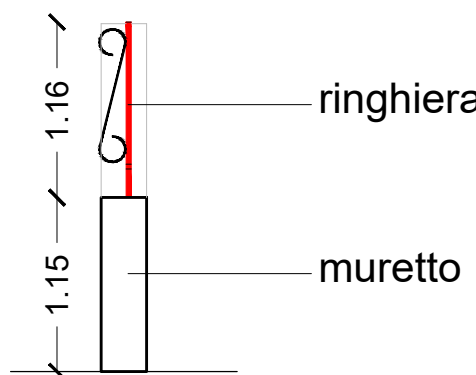
SEZIONE A-A'
