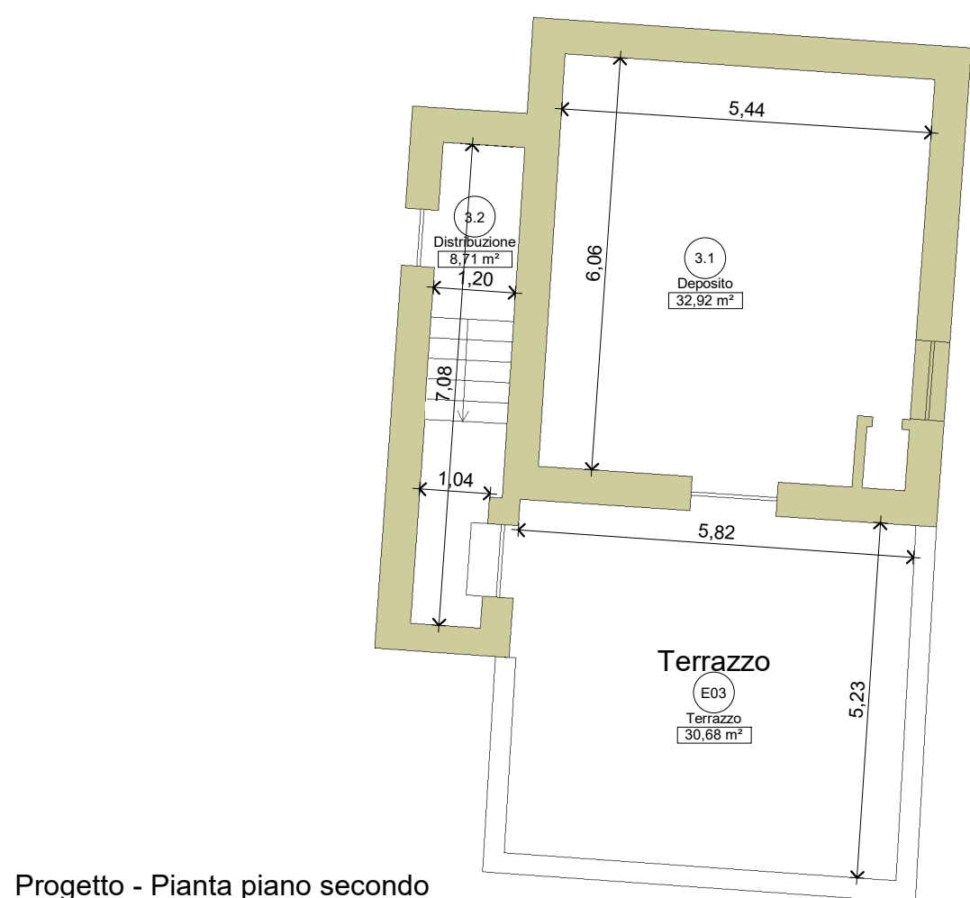
Progetto - Pianta piano secondo Scale 1 : 100
