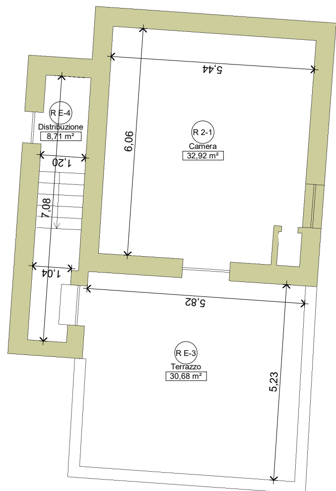
Stato di fatto - piano secondo
